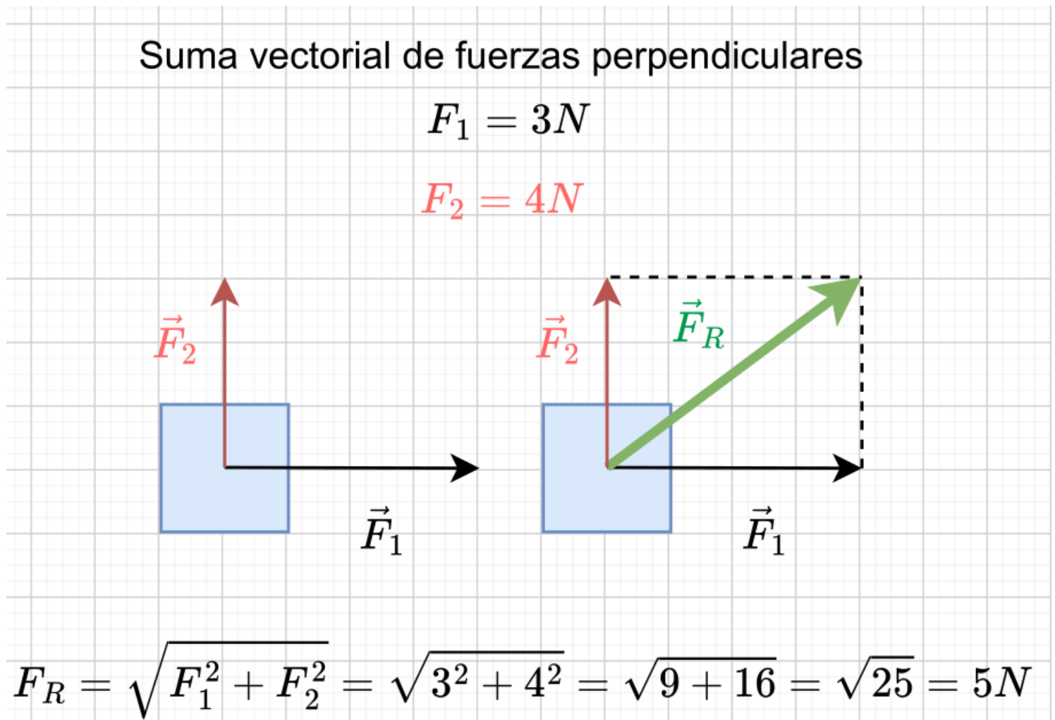
Figura 9: Suma de fuerzas perpendiculares
